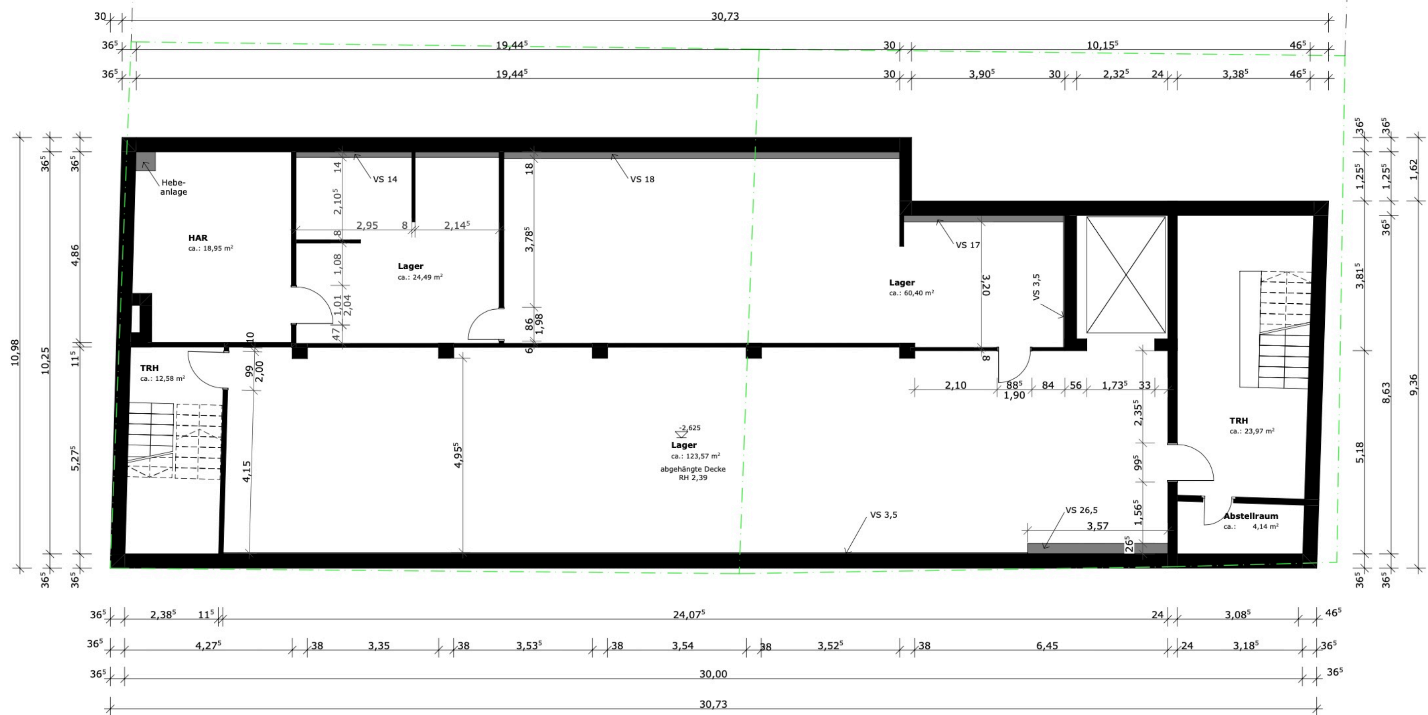
Grundriss Kellergeschoss
