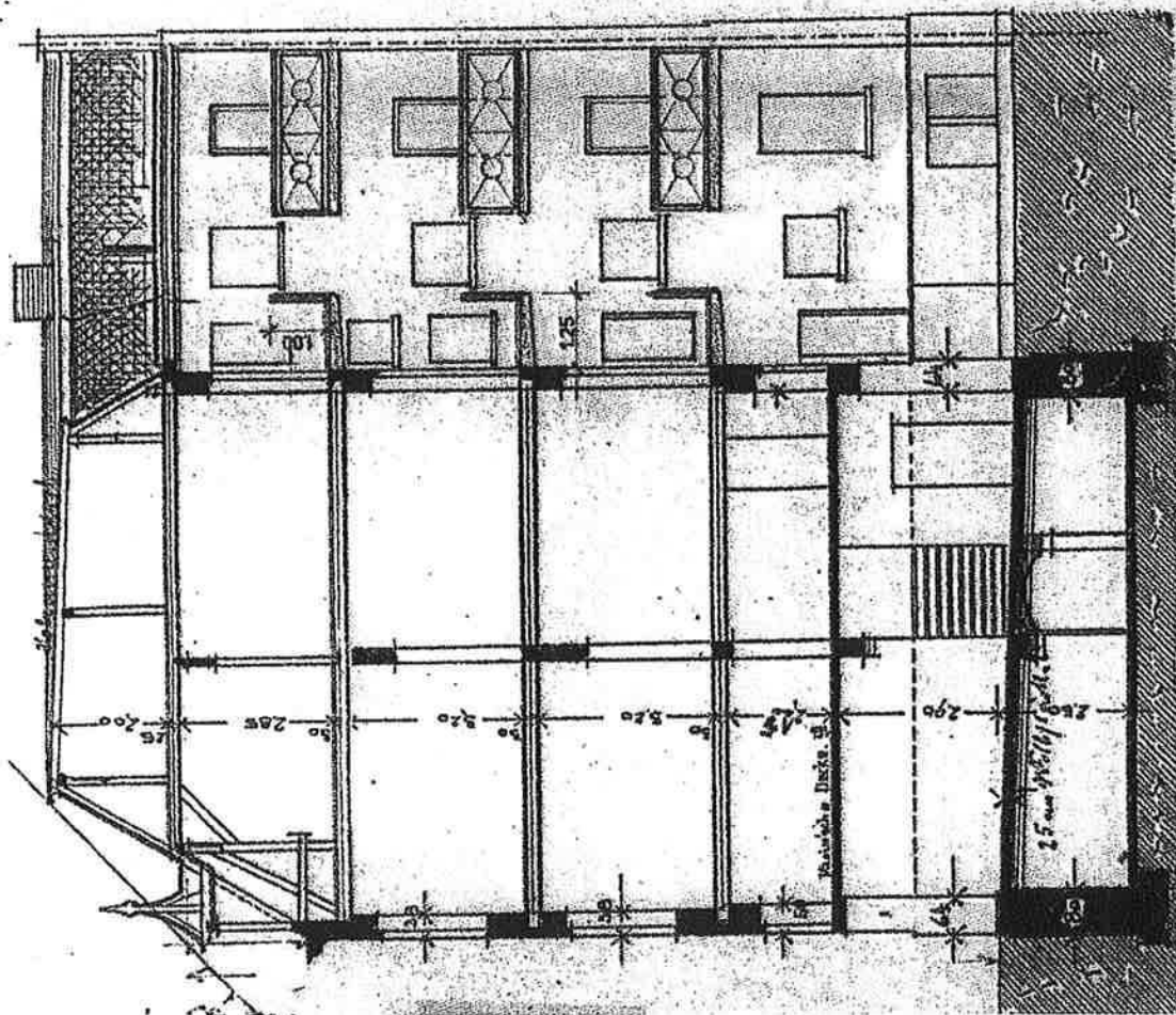
SCHNITT A-B/ANSICHT
