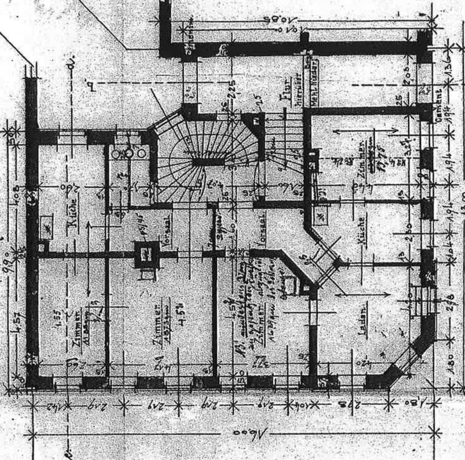
Schnitt c.d.
