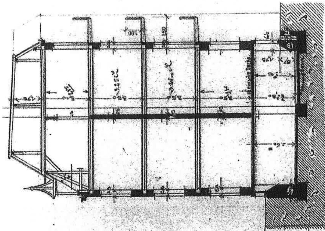
SCHNITT C-D
