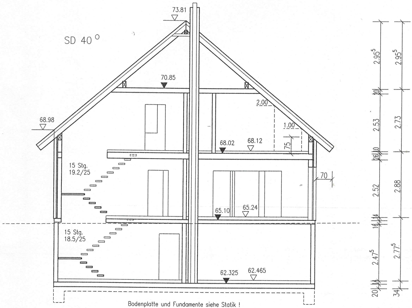
Schnitt A-A
