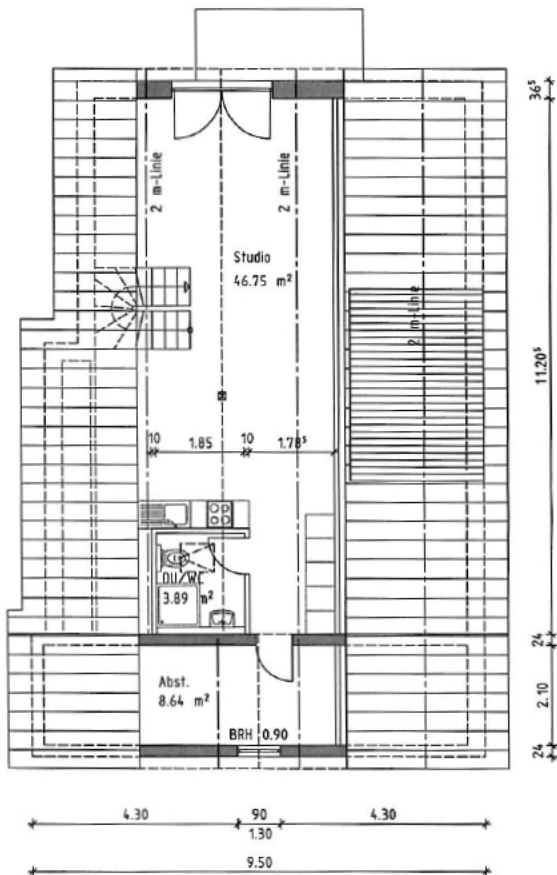
Grundriss Dachgeschoss
