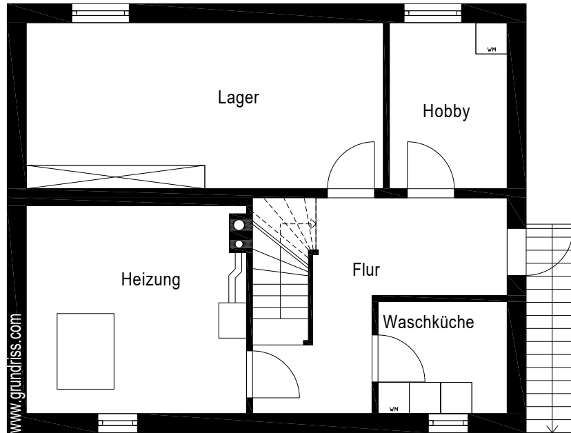
Kellergeschoss
