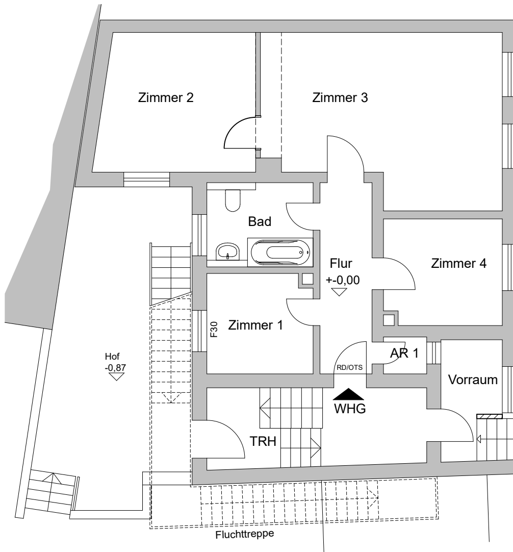
Erdgeschoss M 1:100
