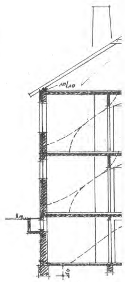
SCHNITT
