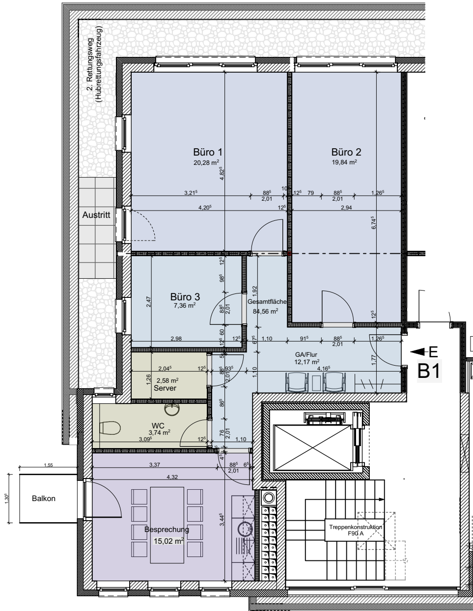
Grundriss Staffelgeschoss Büro_1
