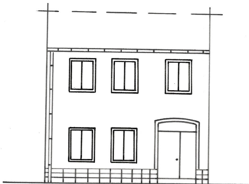
STRASSENANSICHT - NEU
