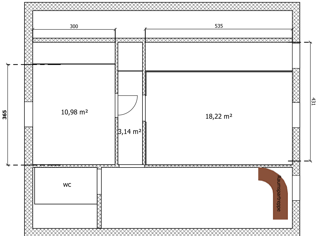
Grundriss Obergeschoss
