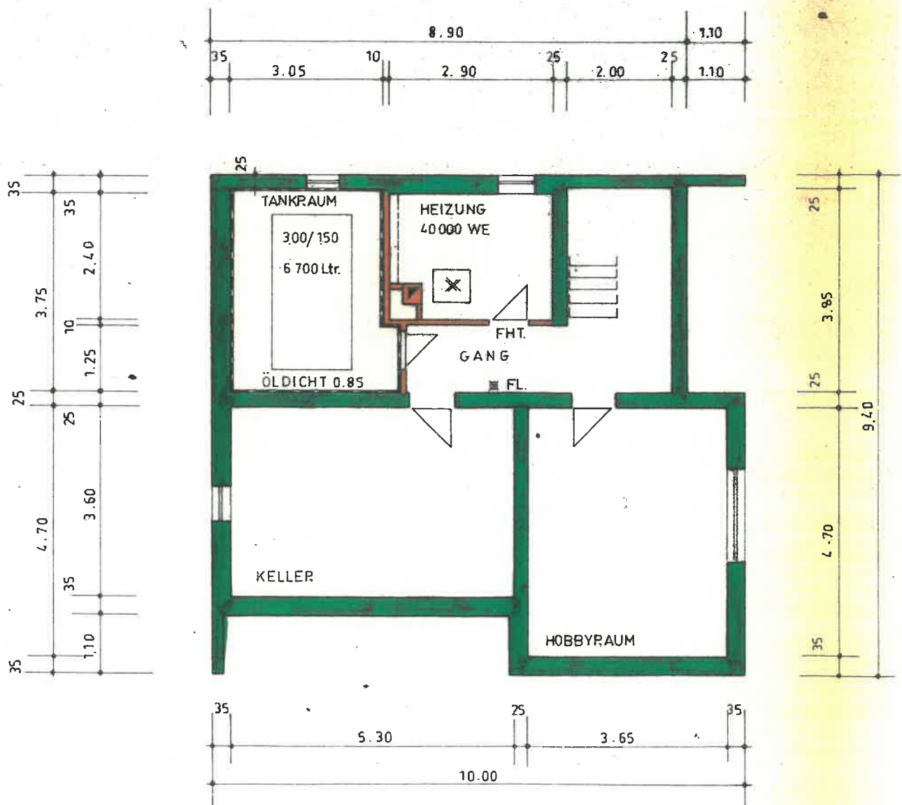
KELLERGESCHOSS
