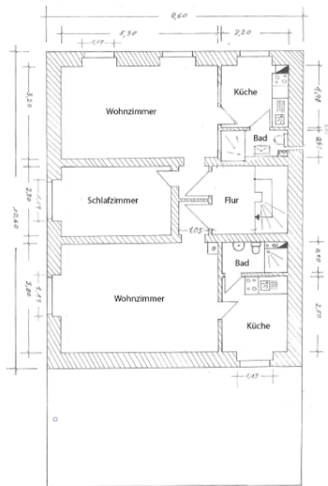
1.OG
