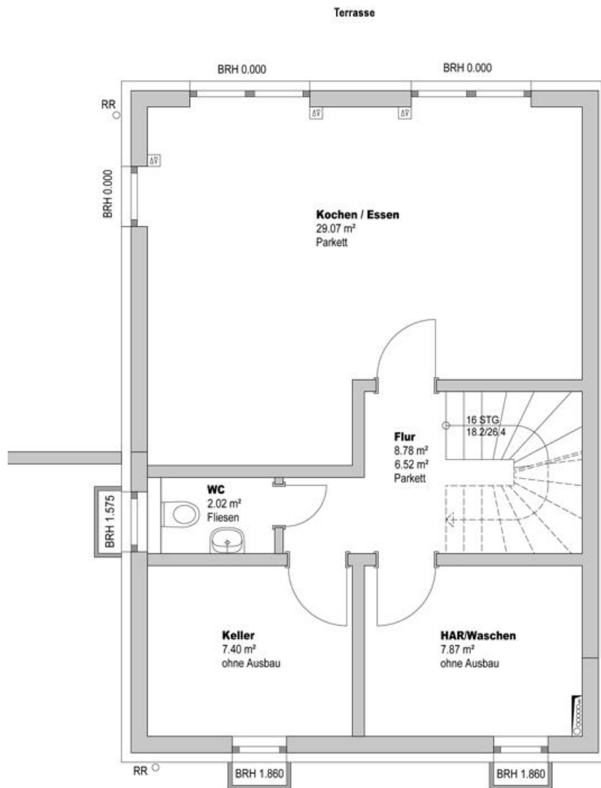
Gartengeschoss
