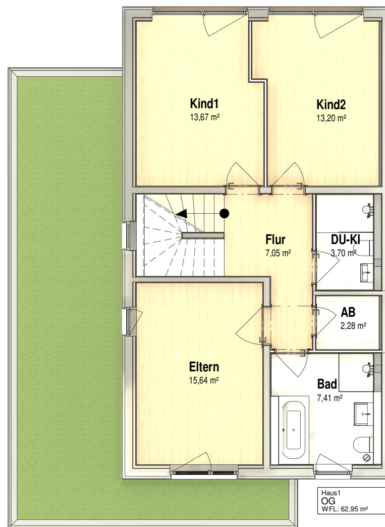
Obergeschoss M 1 : 100
