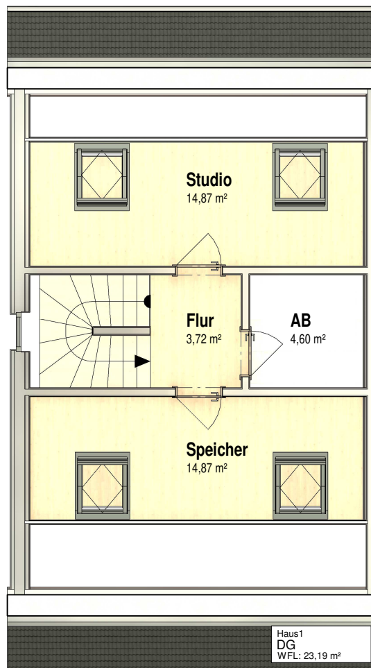
Dachgeschoss M 1 : 100
