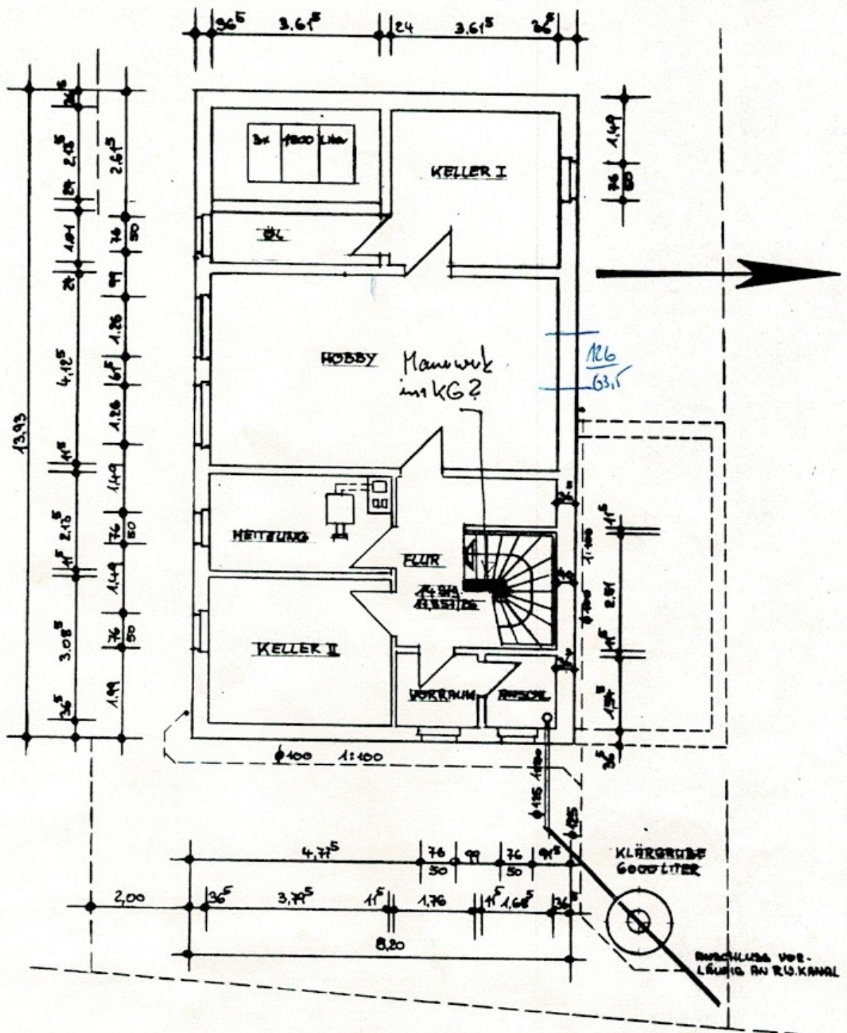
KELLERGESCHOSS M= 1:100
