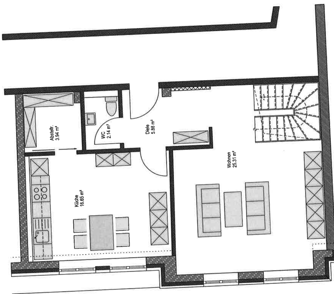
WOHNUNG 6 4.OBERGESCHOSS
