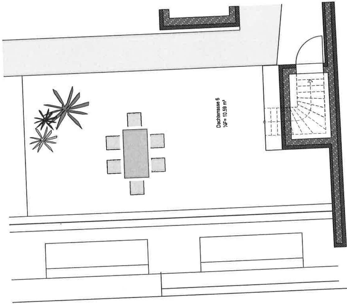
WOHNUNG 6 DACHGESCHOSS
