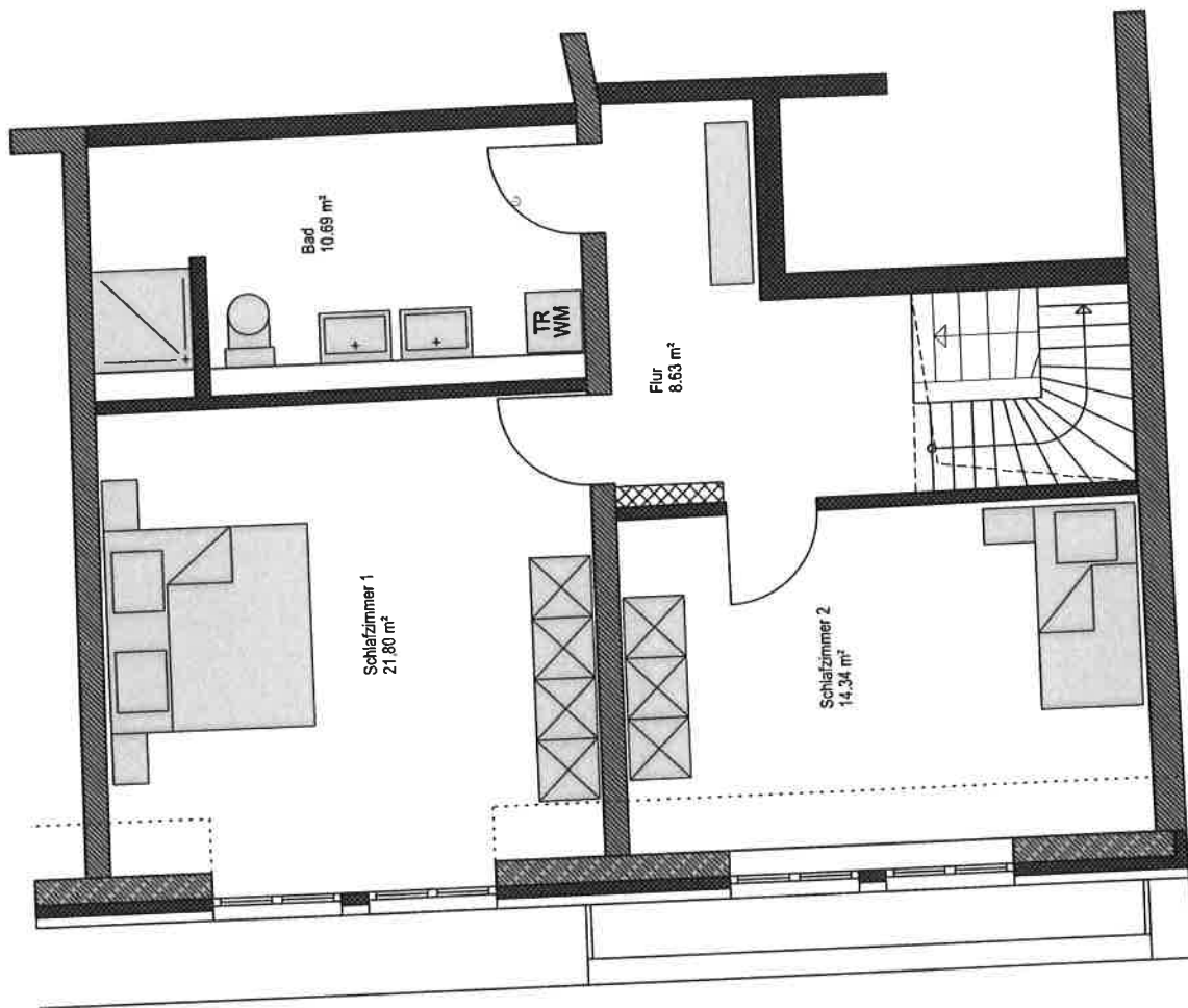
WOHNUNG 6 5.OBERGESCHOSS
