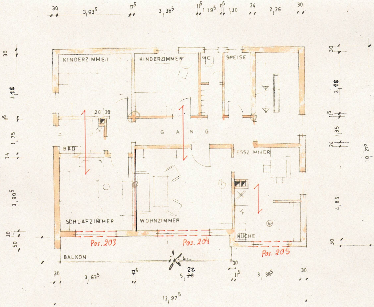
1. OBERGESCHOSS
