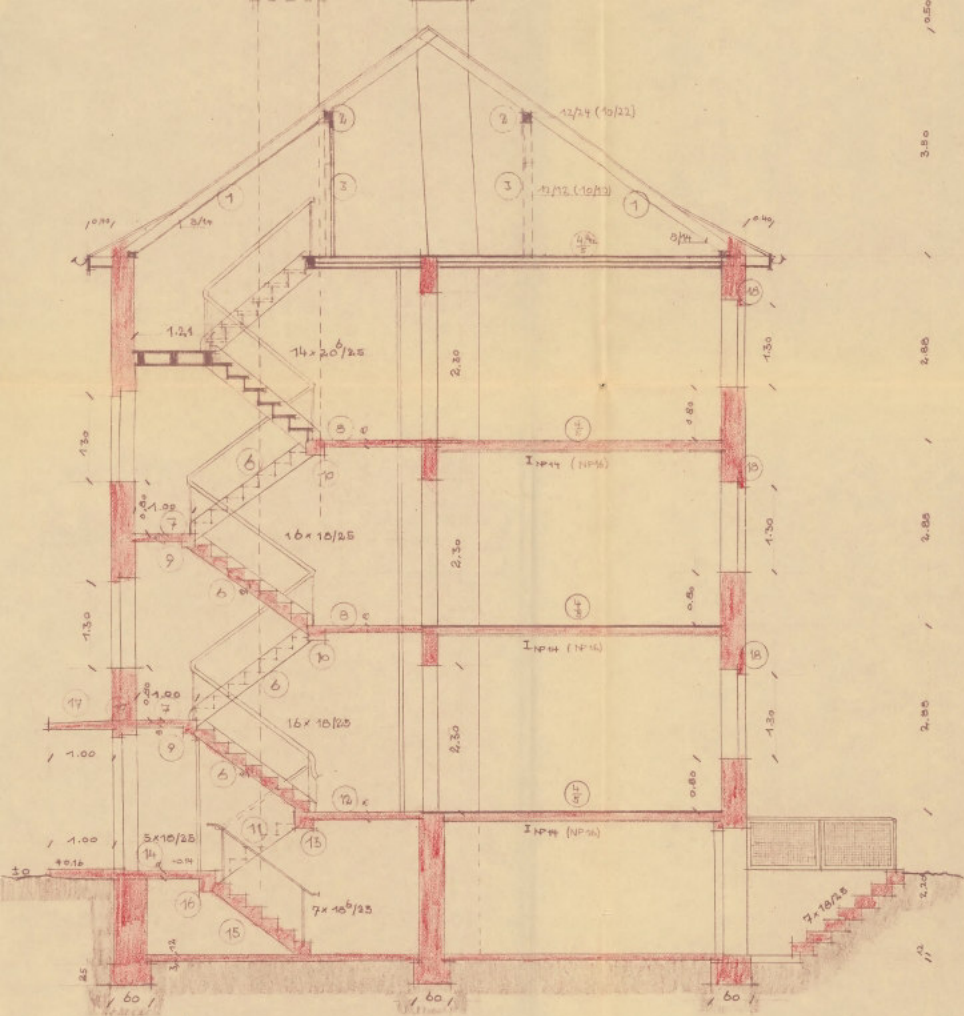
SCHNITT: A-B
