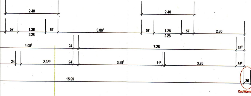
Grundriss DG
