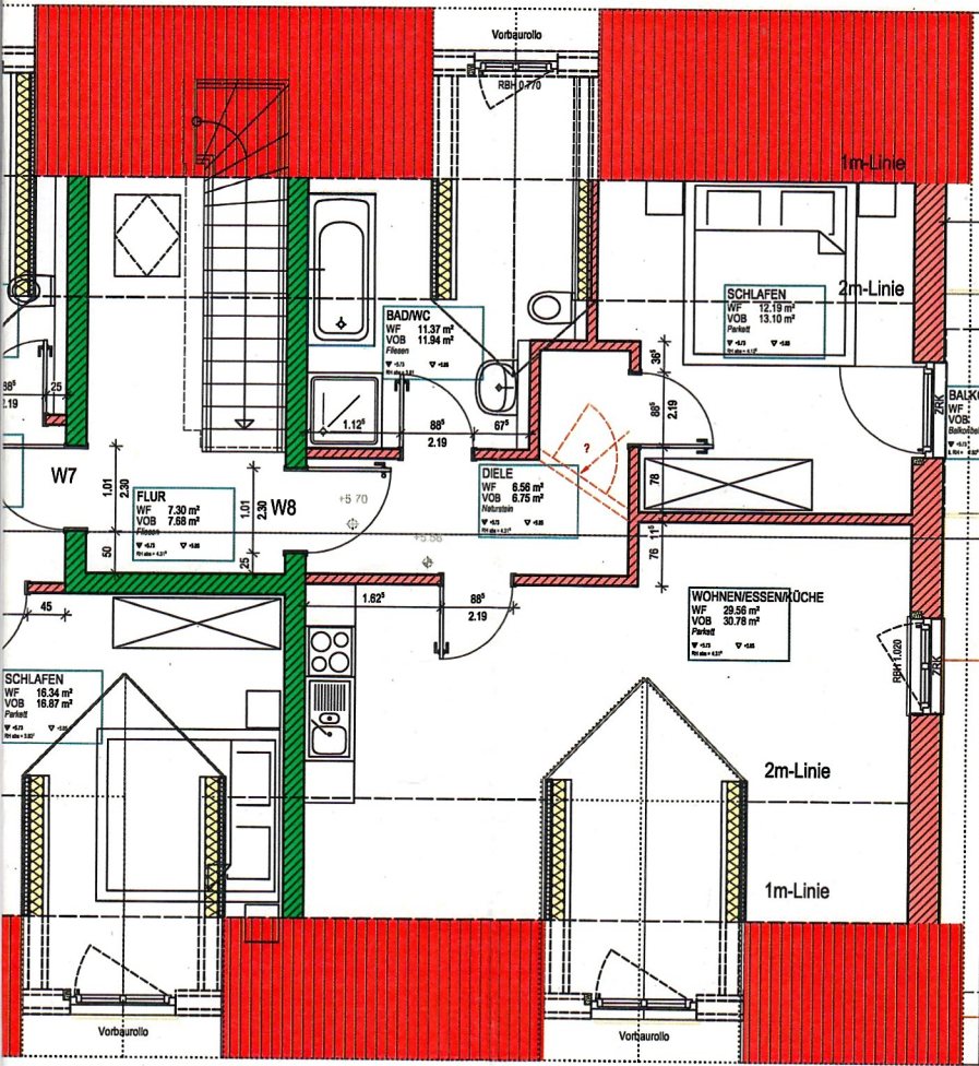
Grundriss DG
