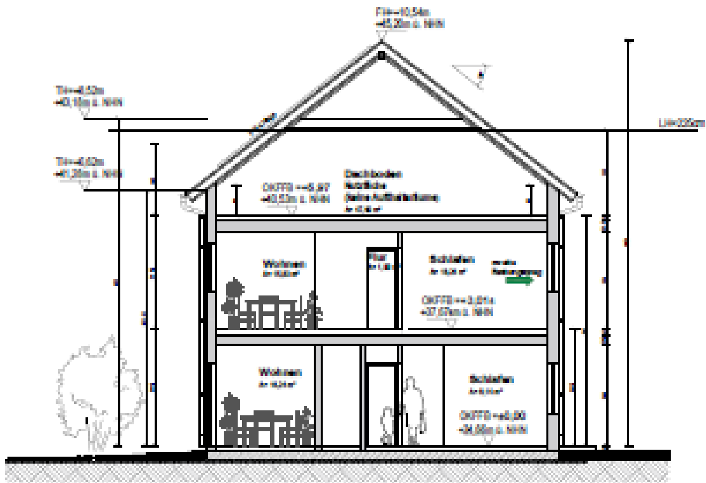
QUERSCHNITT SCHNITT A-A
