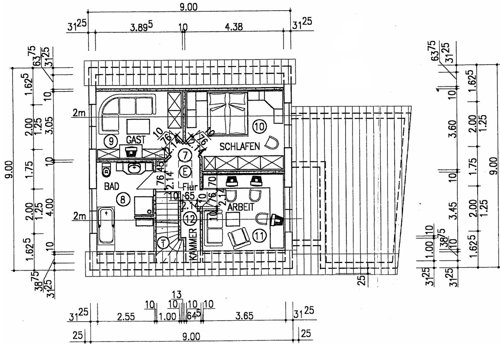
Grundriss Dachgeschoss
