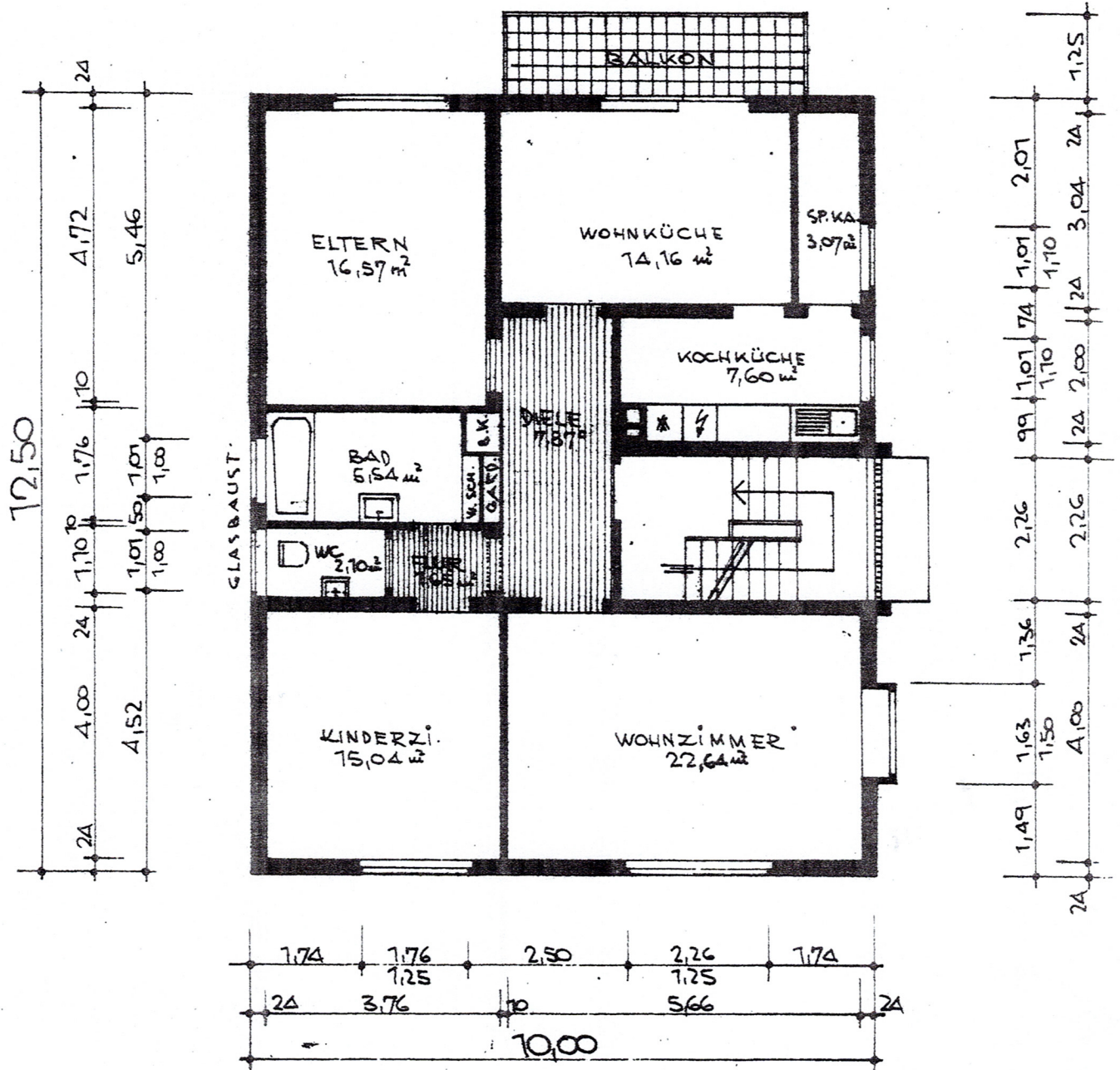
OBERGESCHOSS
