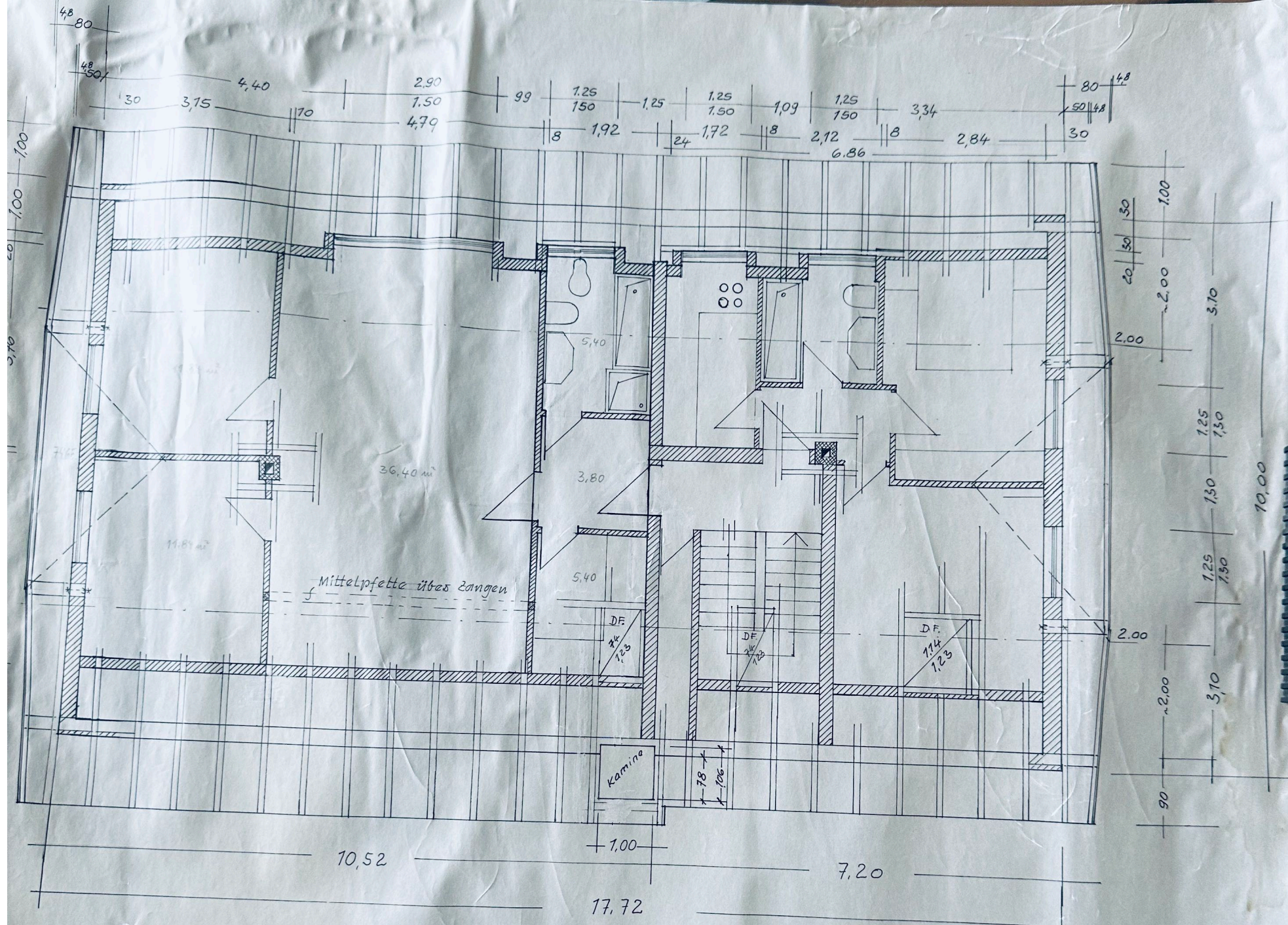
Grundriß Dachgeschoss m. Sparrentagen M=1:50
