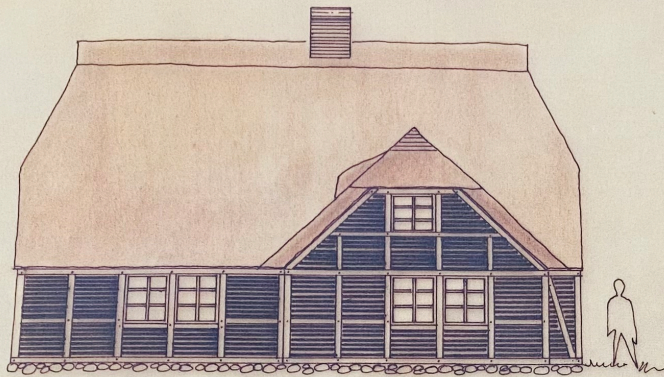
NORDANSICHT
