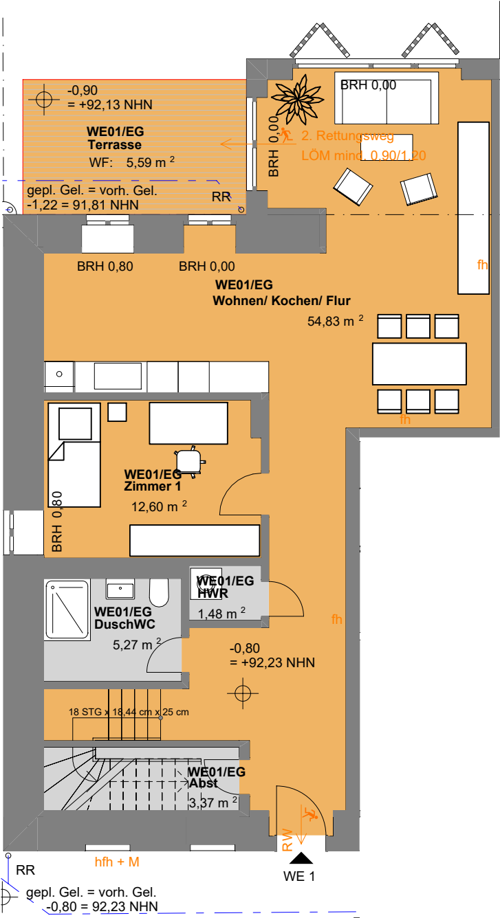
Wohnung 01 - Erdgeschoss
