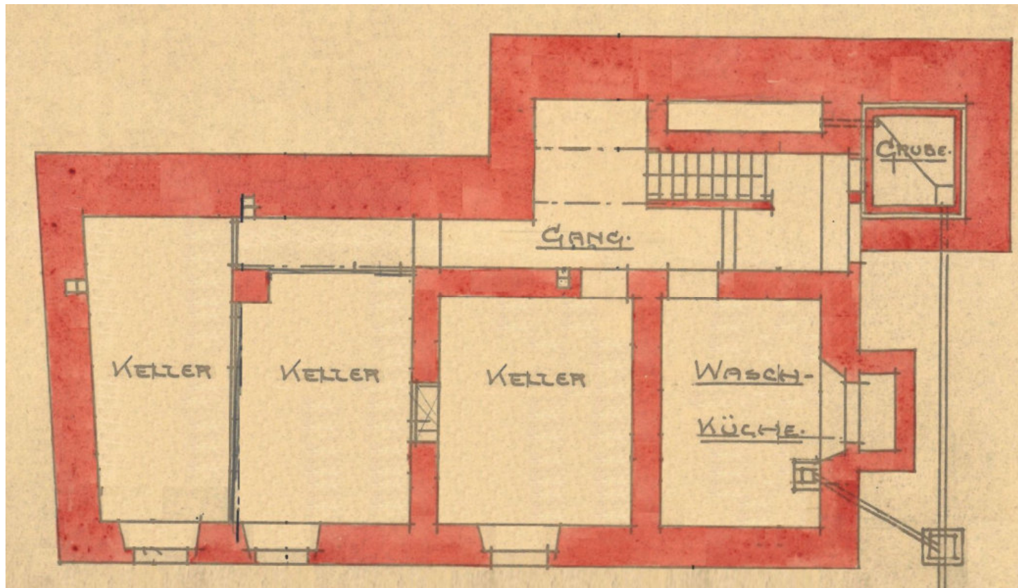
Kellergeschoss
