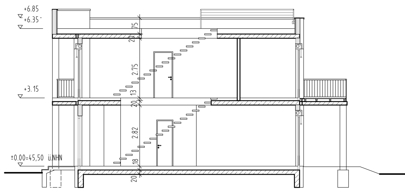
SCHNITT A-A
