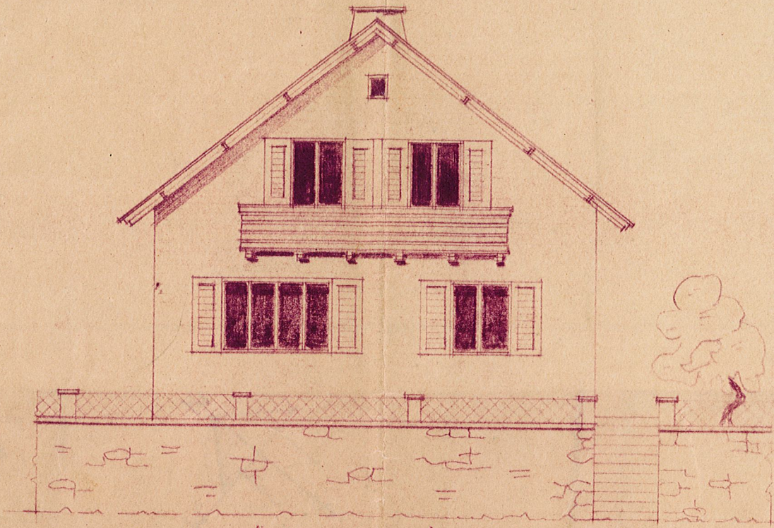
SÜD-WEST-ANSICHT
