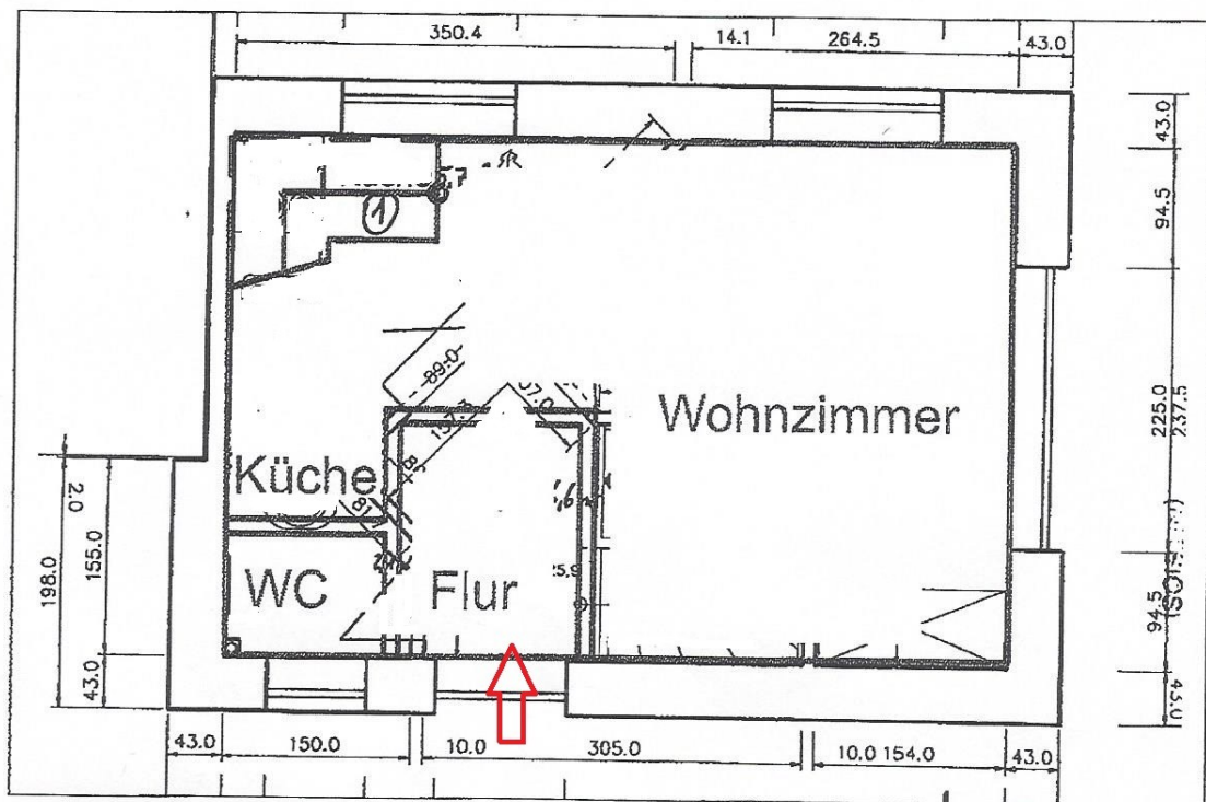
Grundriß Erdgeschoß Anbau
