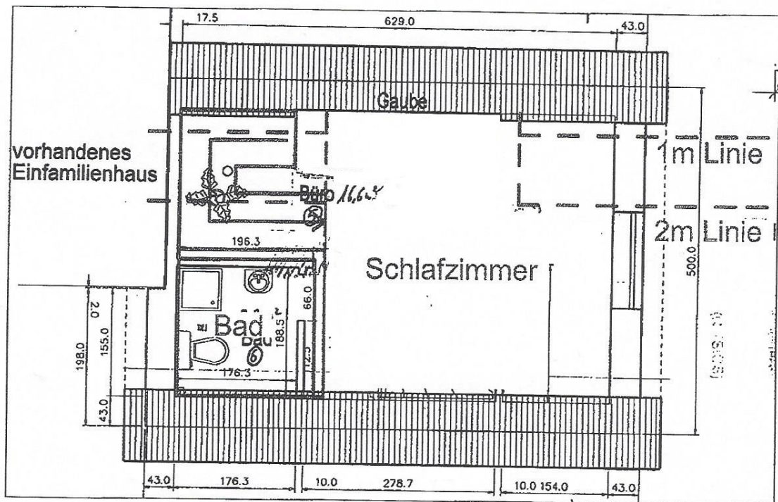
Grundriß Dachgeschoß Anbau
