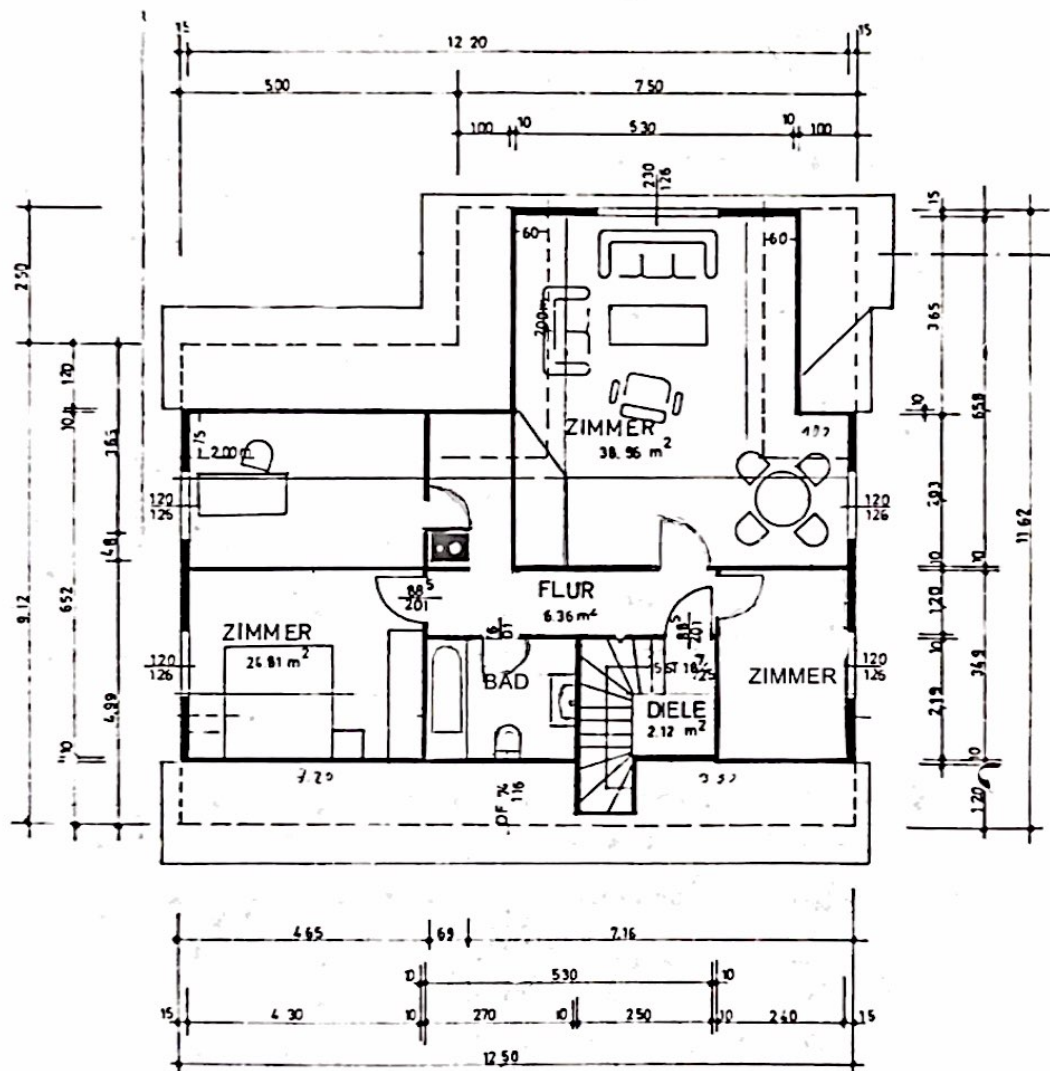
DACHGESCHOSS MERANTIGIEBEL
