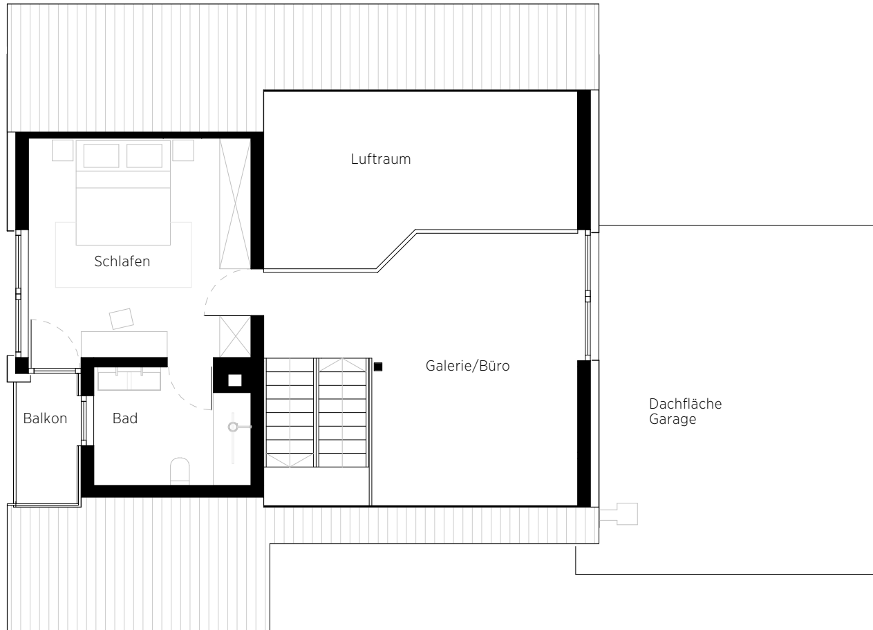
Grundriss OG
