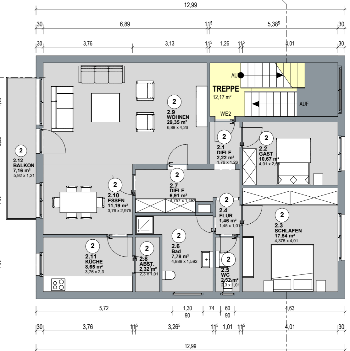
OBERGESCHOSS M 1 : 100
