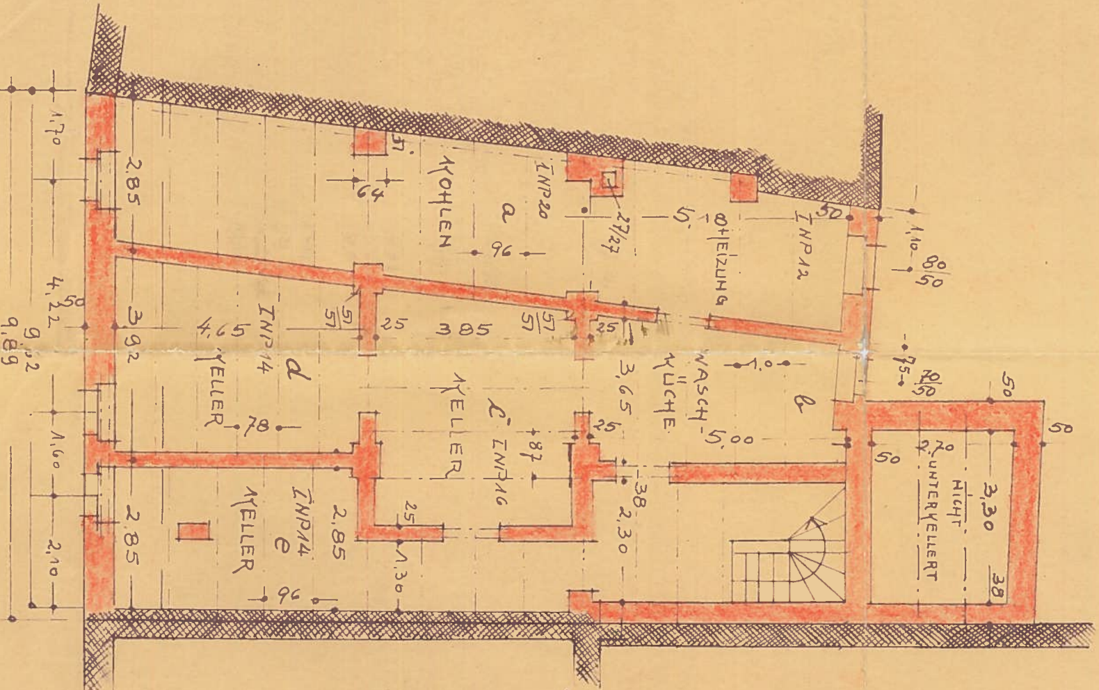
KELLERGESCHOSS
