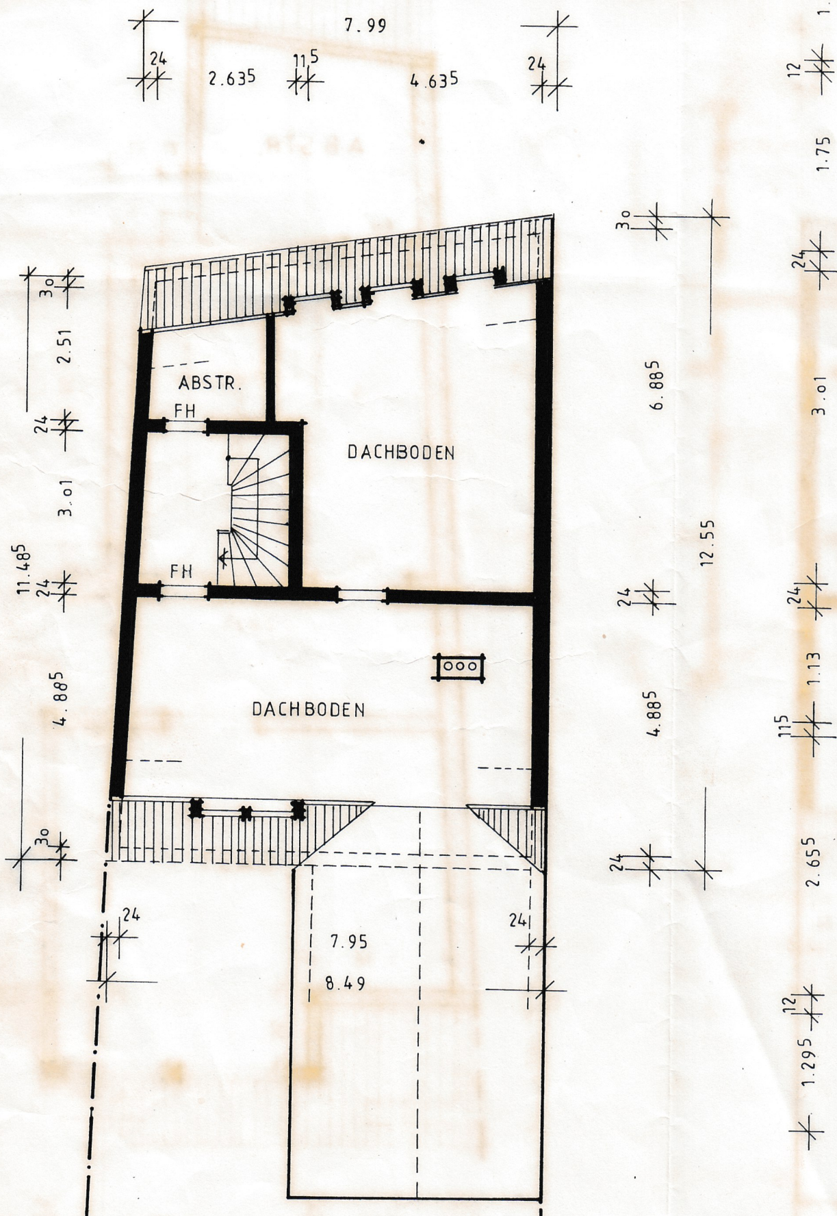
GRUNDRISS D.G. (ALT)
