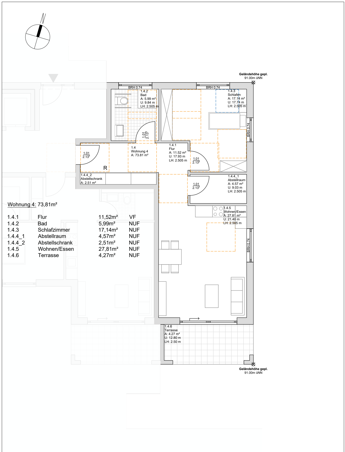
Grundriss Wohnung 4 Neubau Mehrfamilienhaus Von-Emmich Str. 31135 Hildesheim
