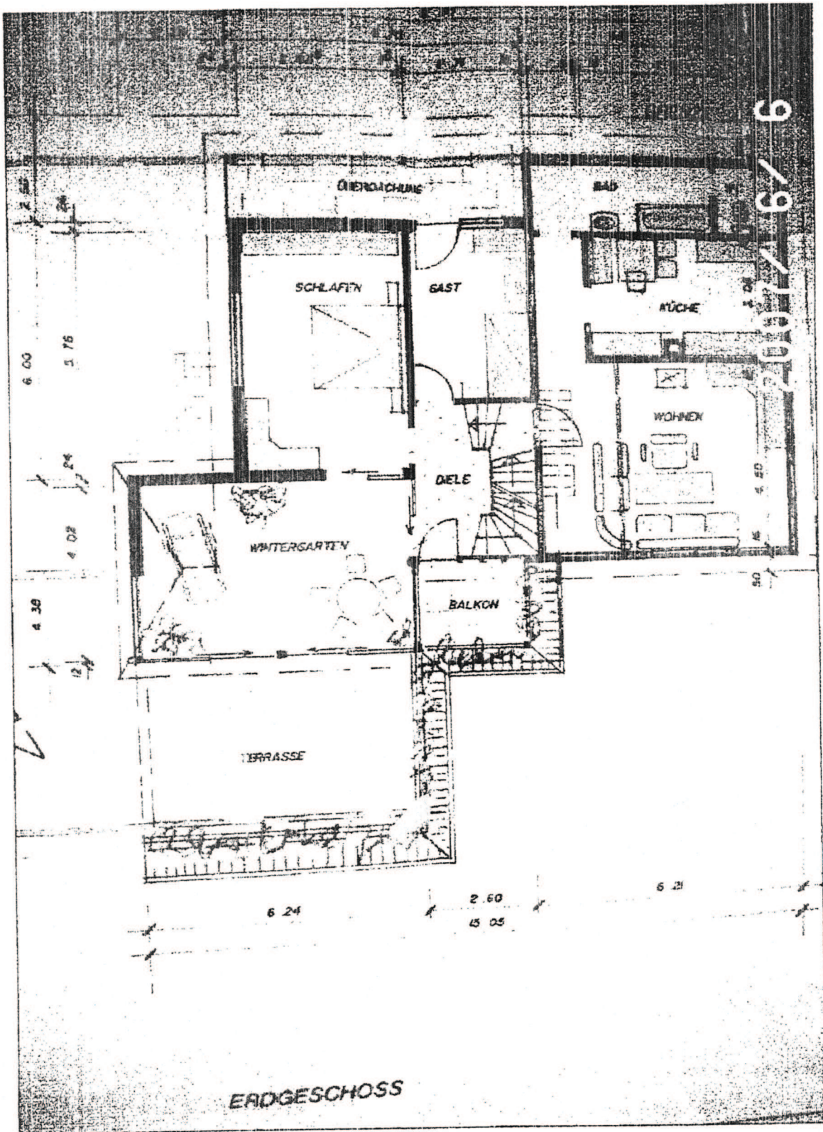
Grundriss Erdgeschoss i.M. 1:100
