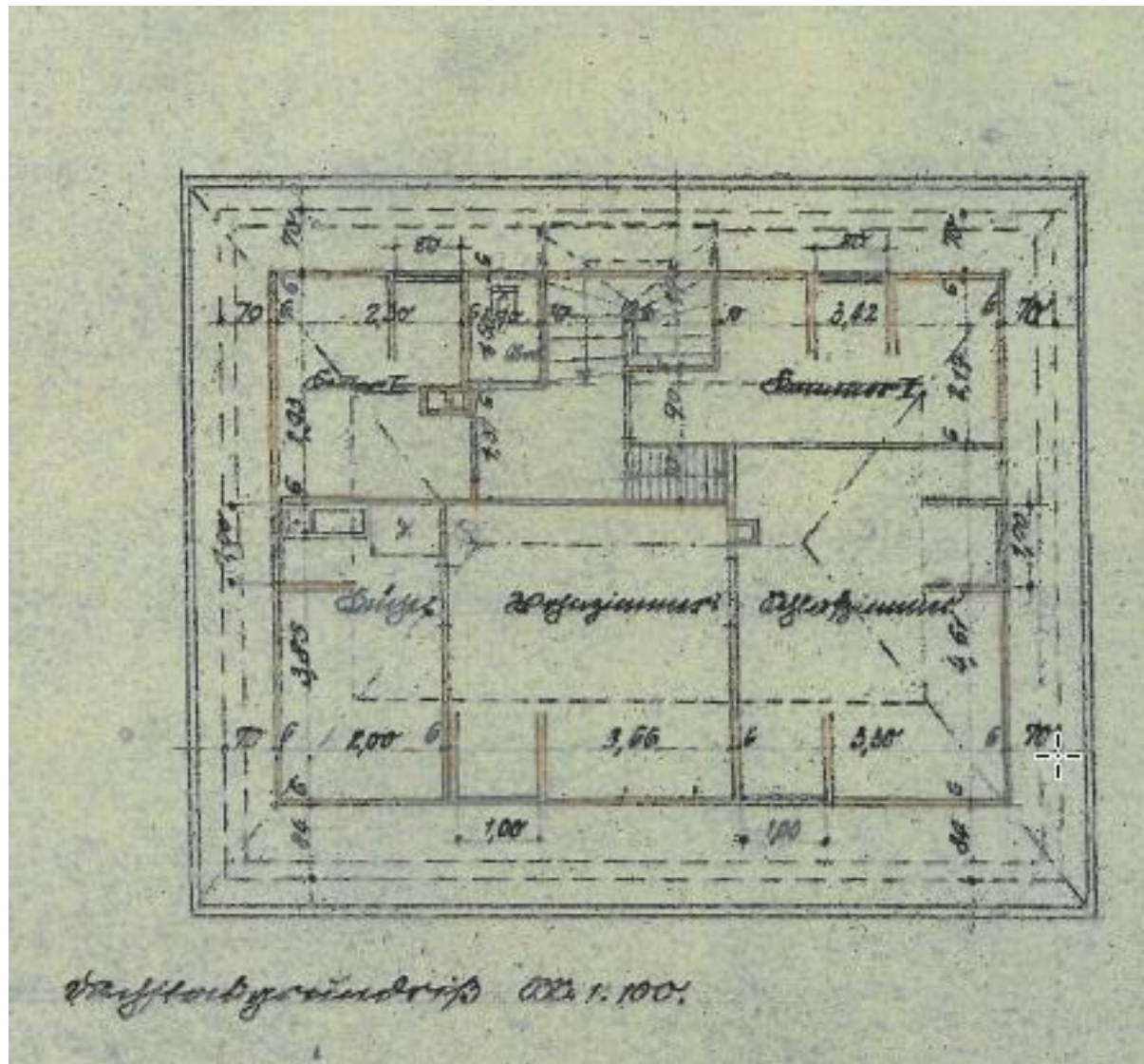
Grundriss-DG-Wohnung:
