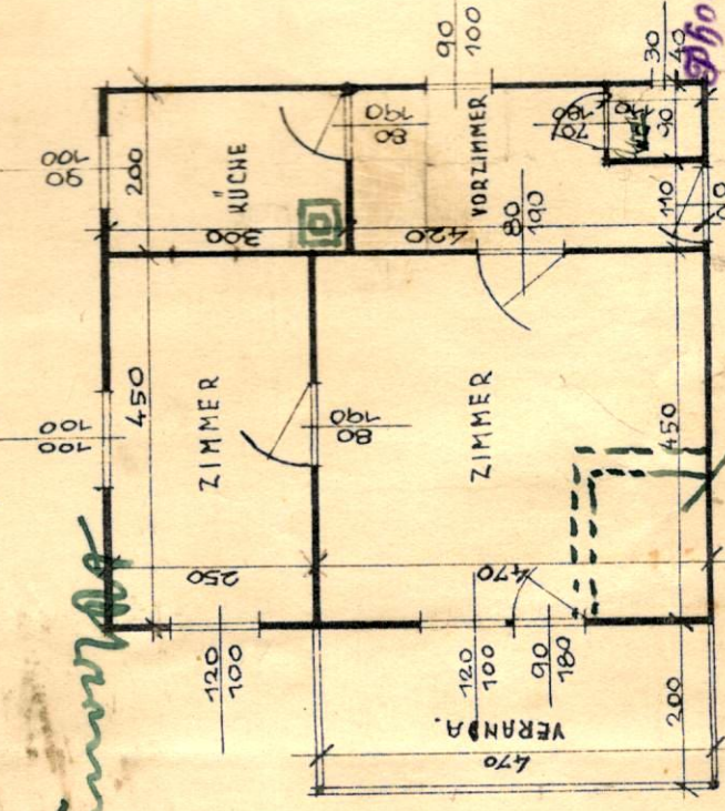
GRUNDRISS.
