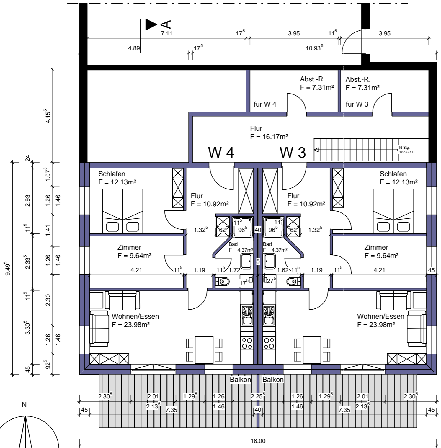
Grundriß Obergeschoss
