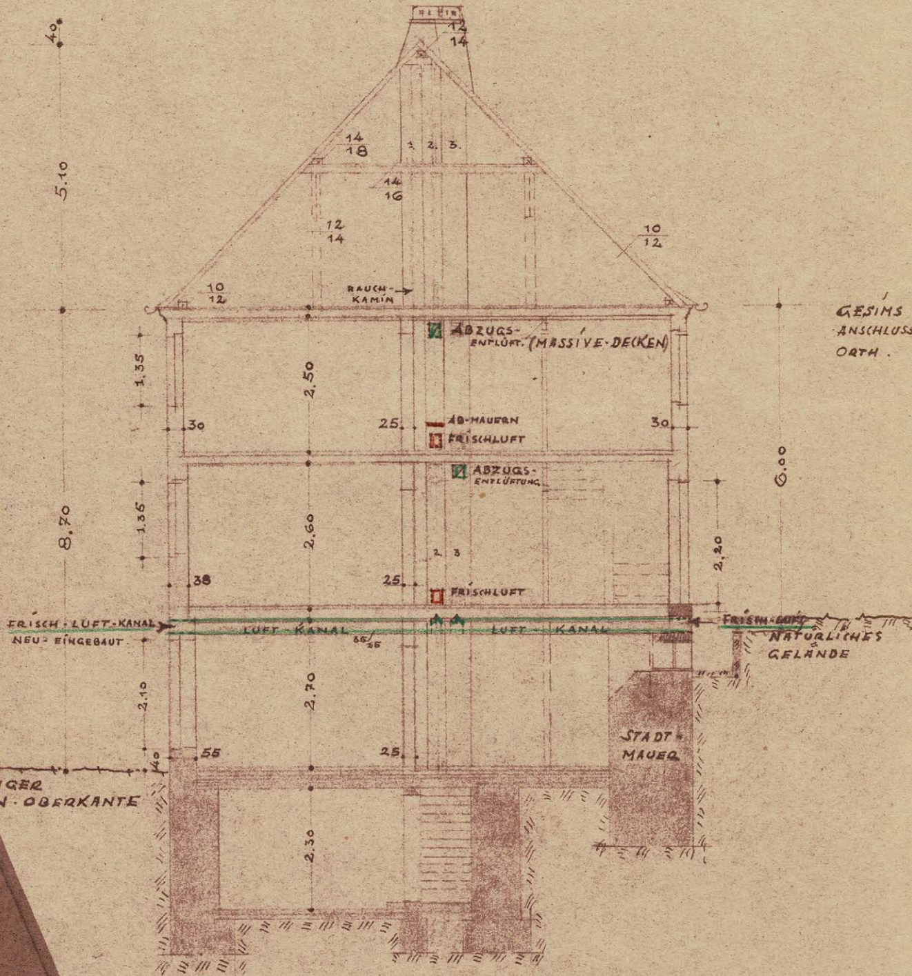
SCHNITT A.-B.
