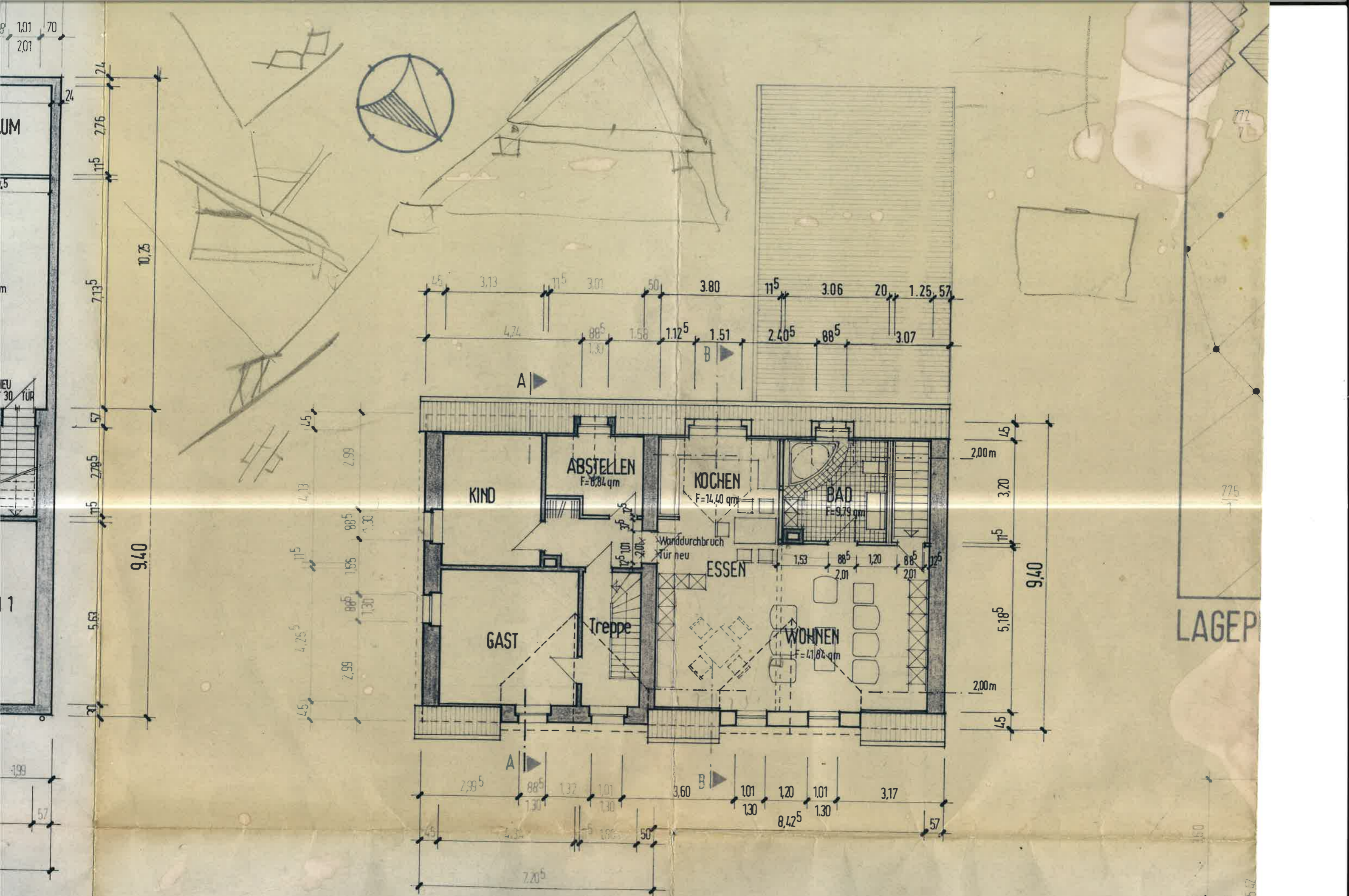
GRUNDRISS DACHGESCHOSS
