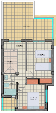
PLANTA ALTA TOP FLOOR
