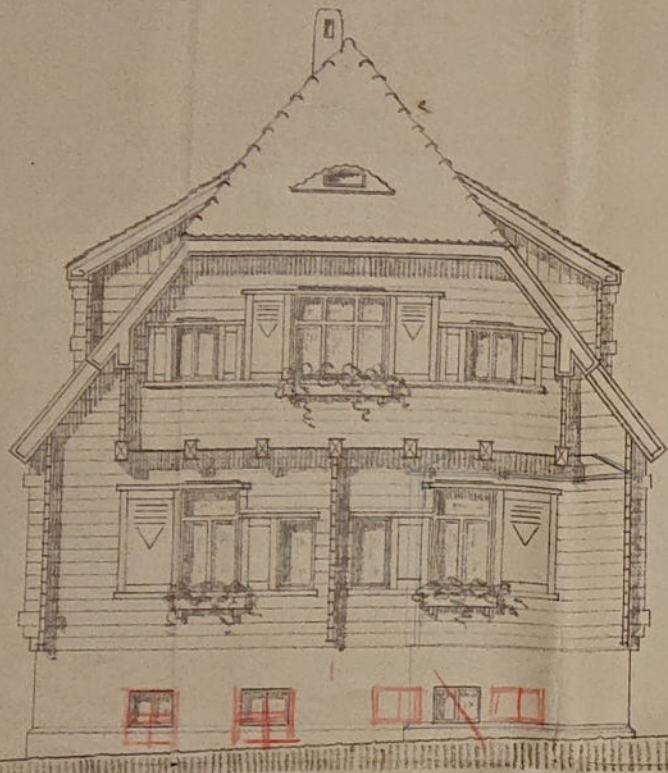
Giebel-Ansicht + Süd-Ost-Frise
