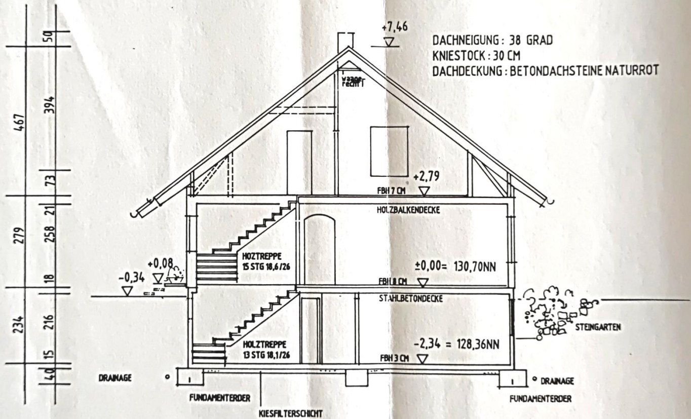
SNITT WOHNHAUS
