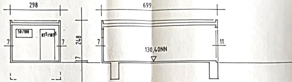
SNITT SCHWÖRER FERTIGGARAGE TYP III
