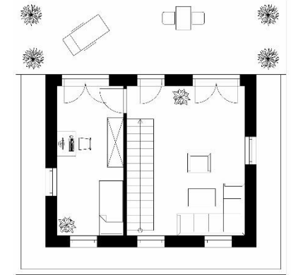
Dachgeschoss
