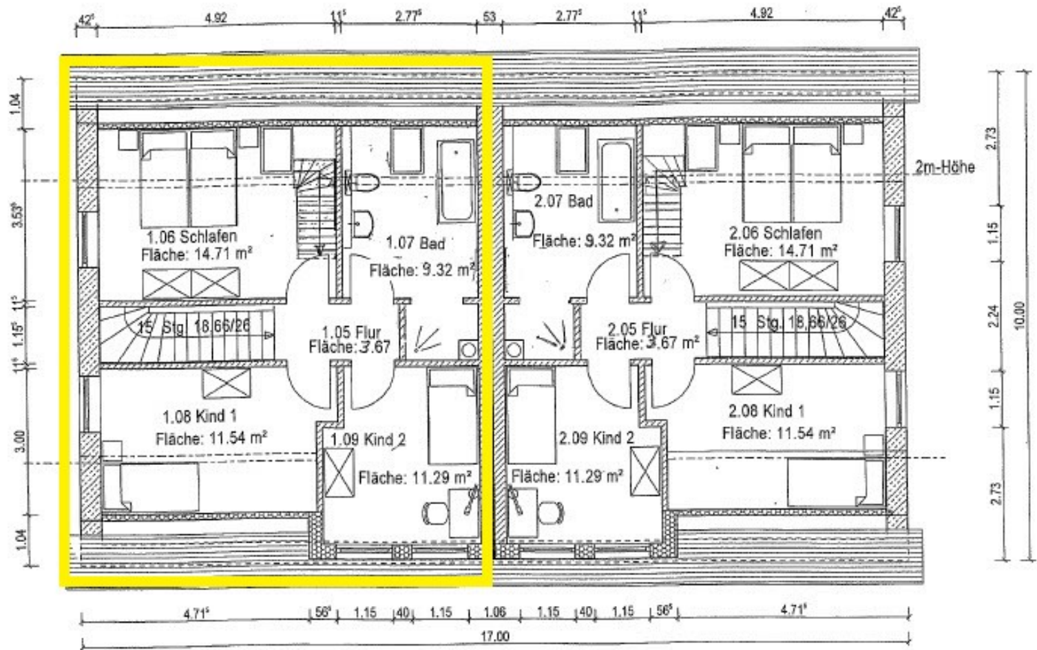
Doppel-Wohnhaus in Seedorf Grundriss - Dachgeschoss
