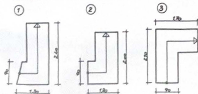
ROHBAU-PLANUNGSSKIZZE FÜR DIE TREPPEN
