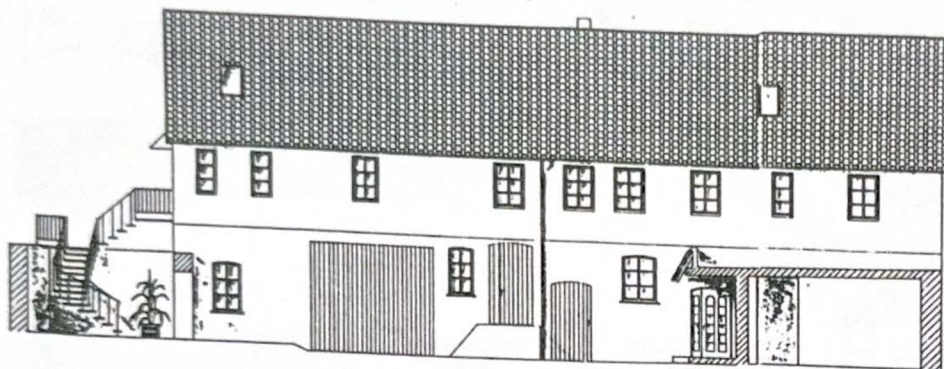
OSTANSICHT (STRASSE)
