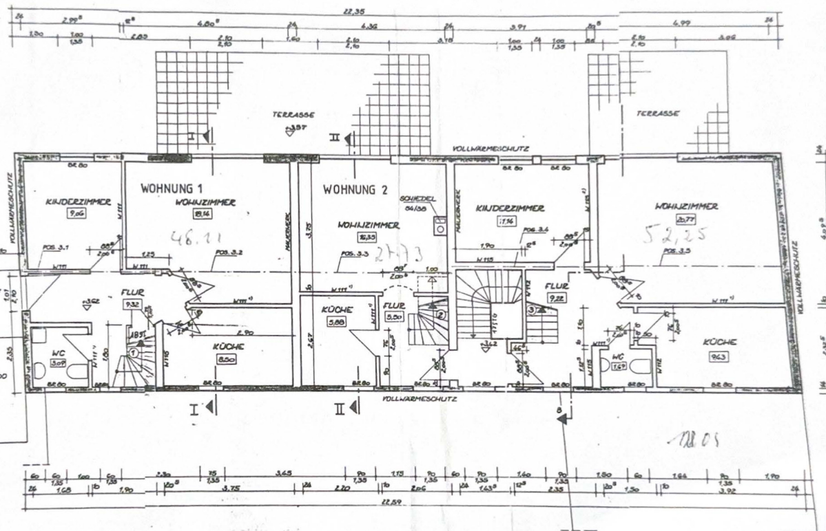
ROHBAU-PLANUNGSSKIZZE FÜR DIE TREPPEN
