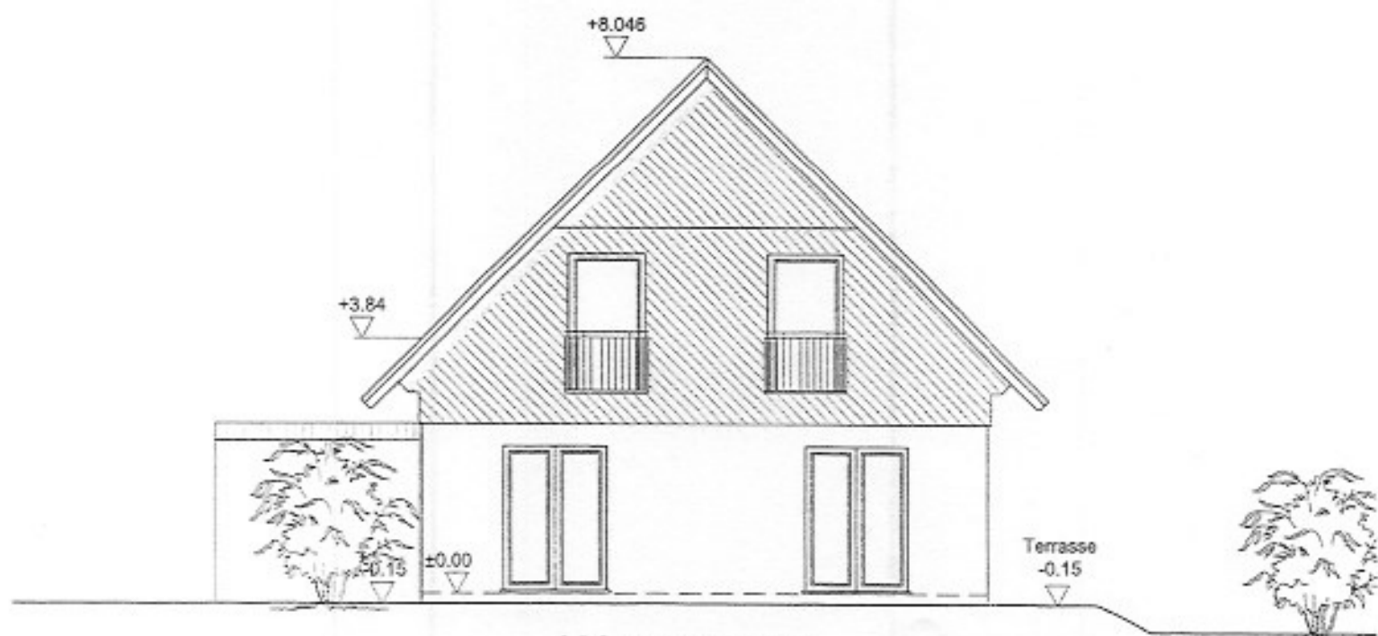
Westansicht Gartenansicht
