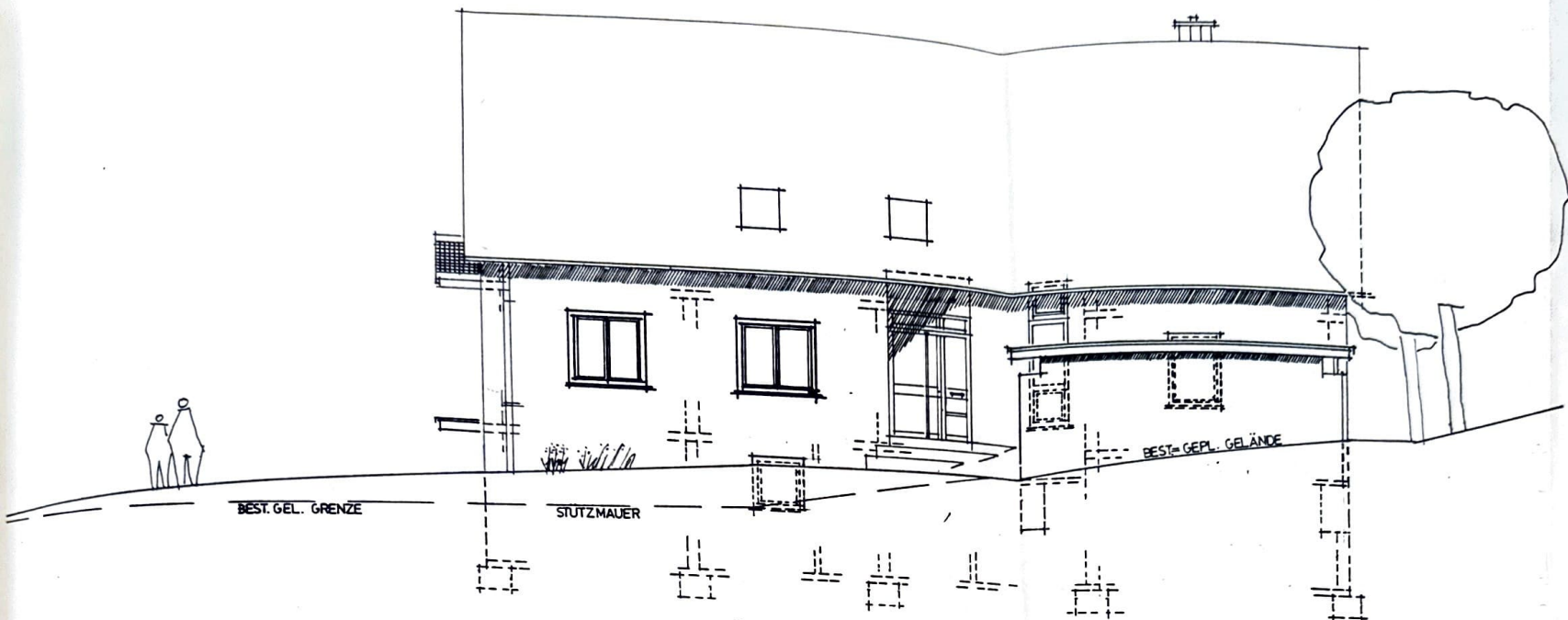
SÜD-OST ANSICHT
