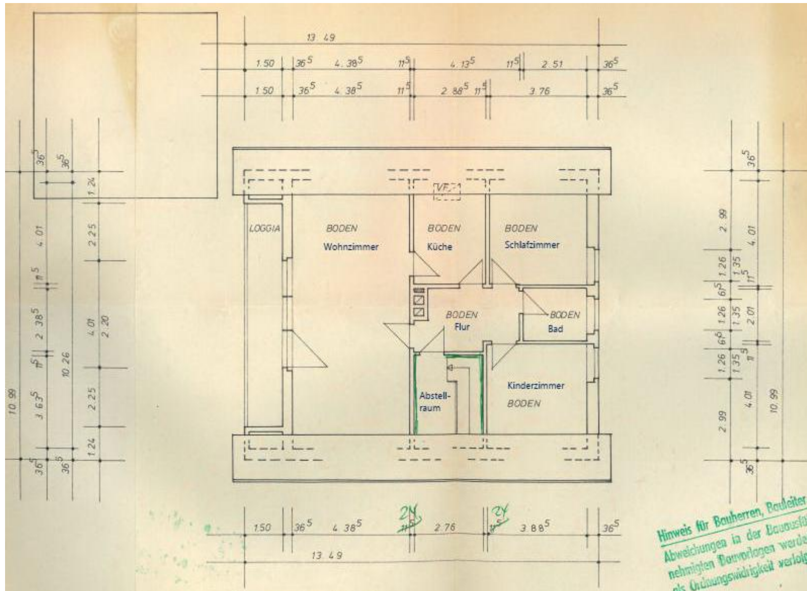
DACHGESCHOSS
